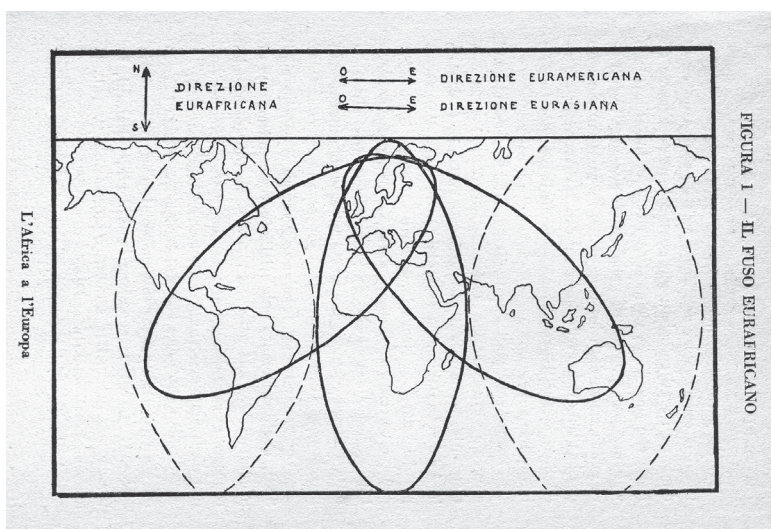
Figure 2.4 Cartographic representation of the three main geopolitical axes, with the Eurafrican axis at the centre. Source: Paolo d'Agostini Orsini di Camerota, Eurafrica: L'Africa per l'Europa, l'Europa per l'Africa (Rome: Paolo Cremonese, 1934).
